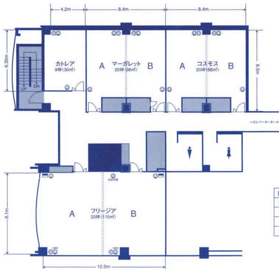
5階 小宴会場「フリージア」・「コスモス」 「マーガレット」・「カトレア」平面図 天井高 2.7m
